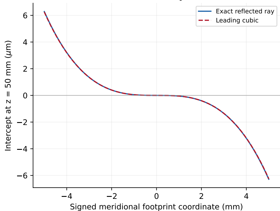
Transverse ray fan
